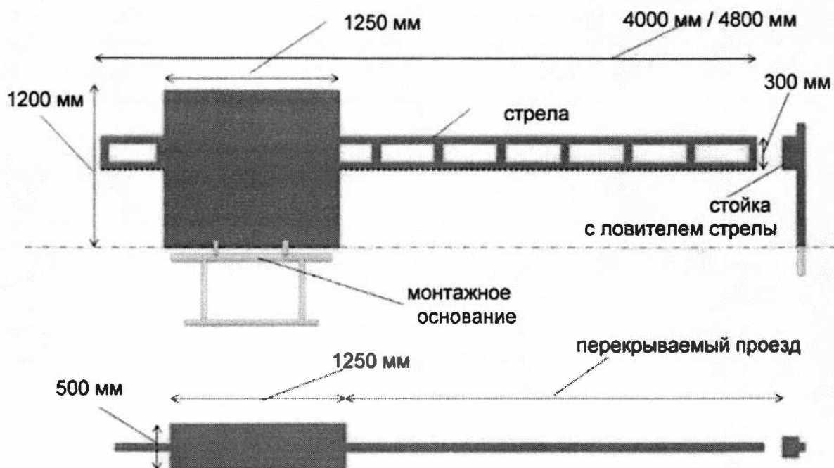
Рис. 3. Размеры шлагбаума
